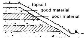
4 Layered fill
